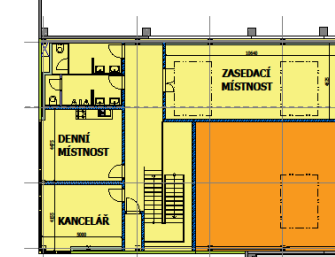
2.NP - 176 m 2
